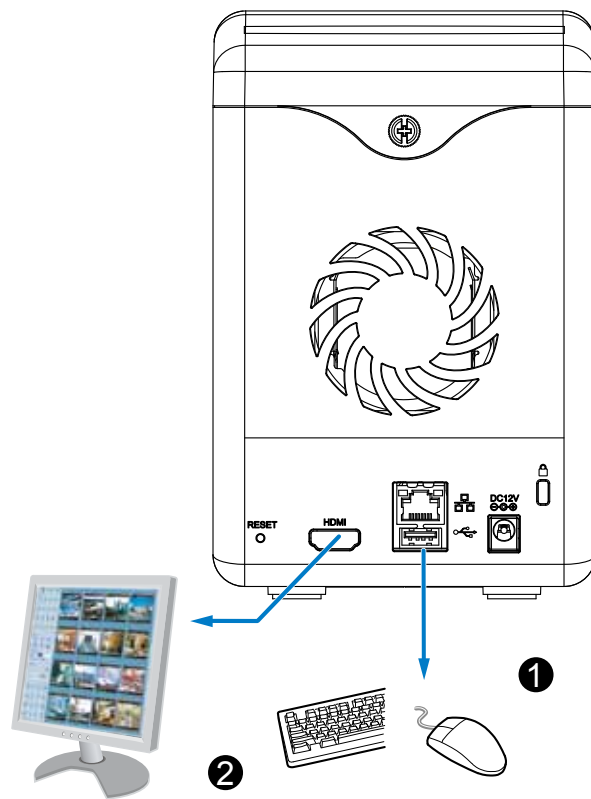
Local console
